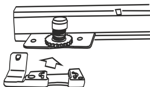
Правая направляющая
