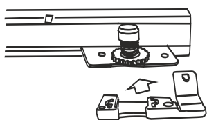
Левая направляющая
