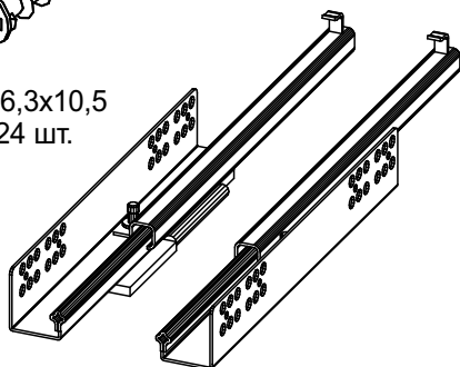
Направляющие L=400 мм - 6 к-та
